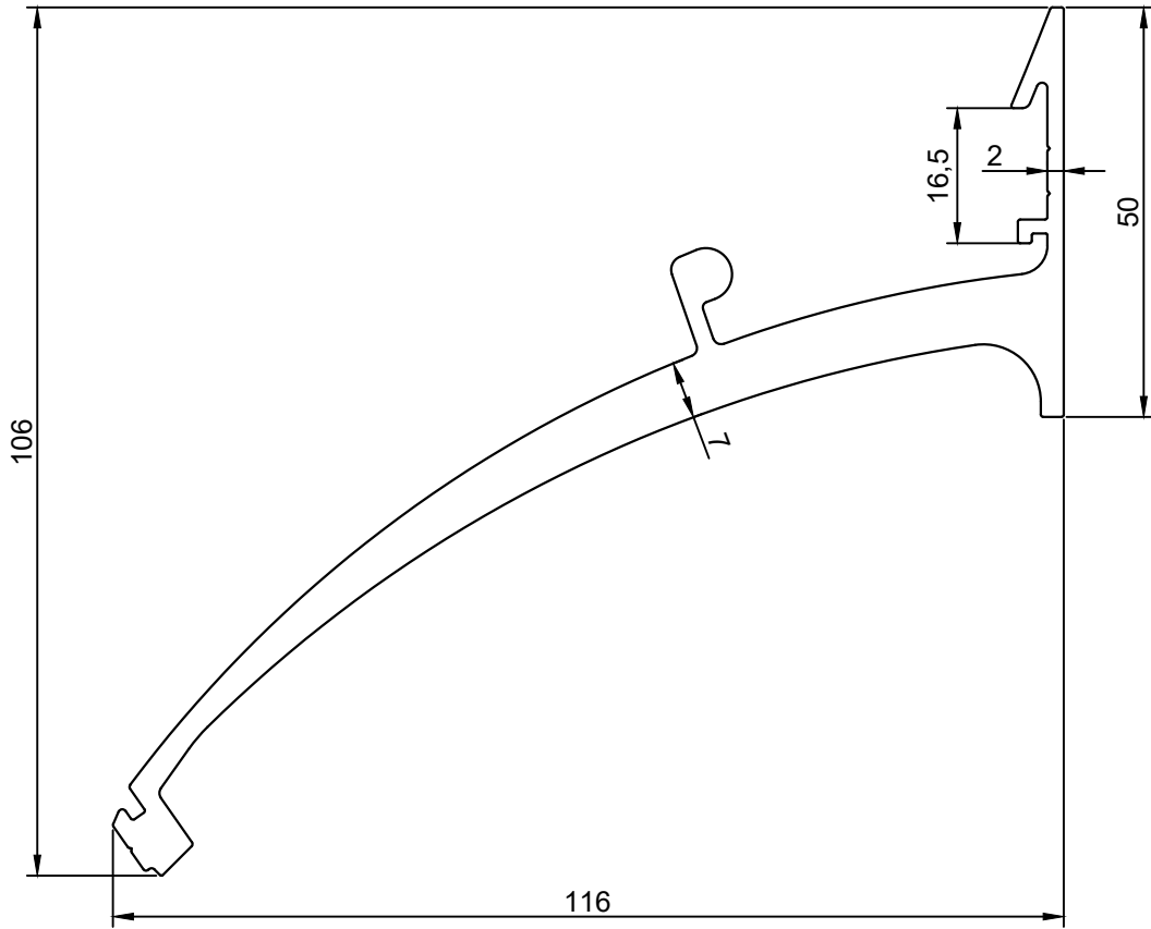
Profil No: 1117 Ağırlık : 2,746 Kg/m
