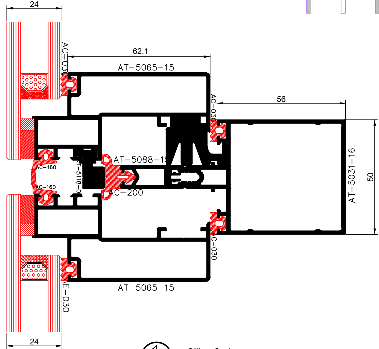
Silikon Cephe Palalet Kaset Detayı
