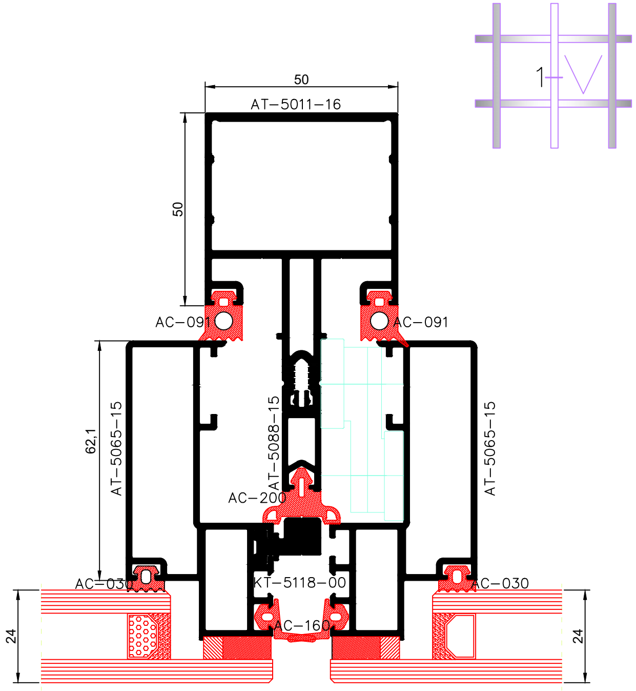
Silikon Cephe Palalel Kaset - Gizli Kanat Detayı
