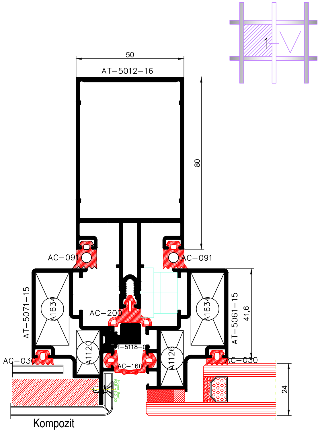
Silikon Cephe Kasetli Kompozit Detayı
