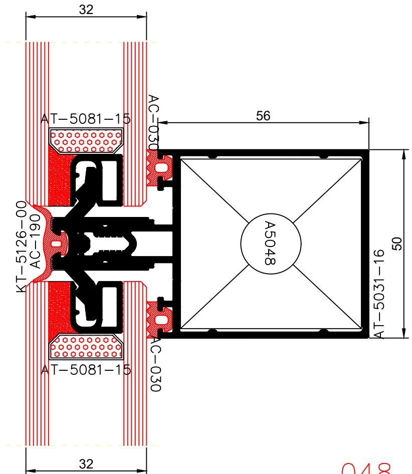
Silikon Cephe Cam Klipsi Detayı
