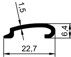
Profil No: 1118 Ağırlık : 0,125 Kg/m
