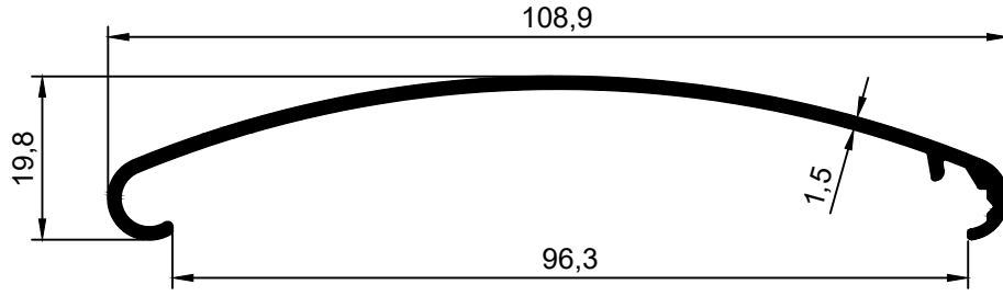
Profil No: 1116 Ağırlık : 0,554 Kg/m
