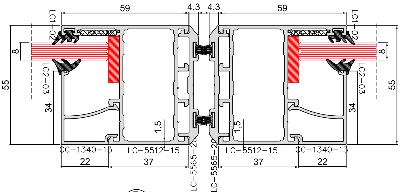
Dar Çarpma Kapı Kilit Detay
