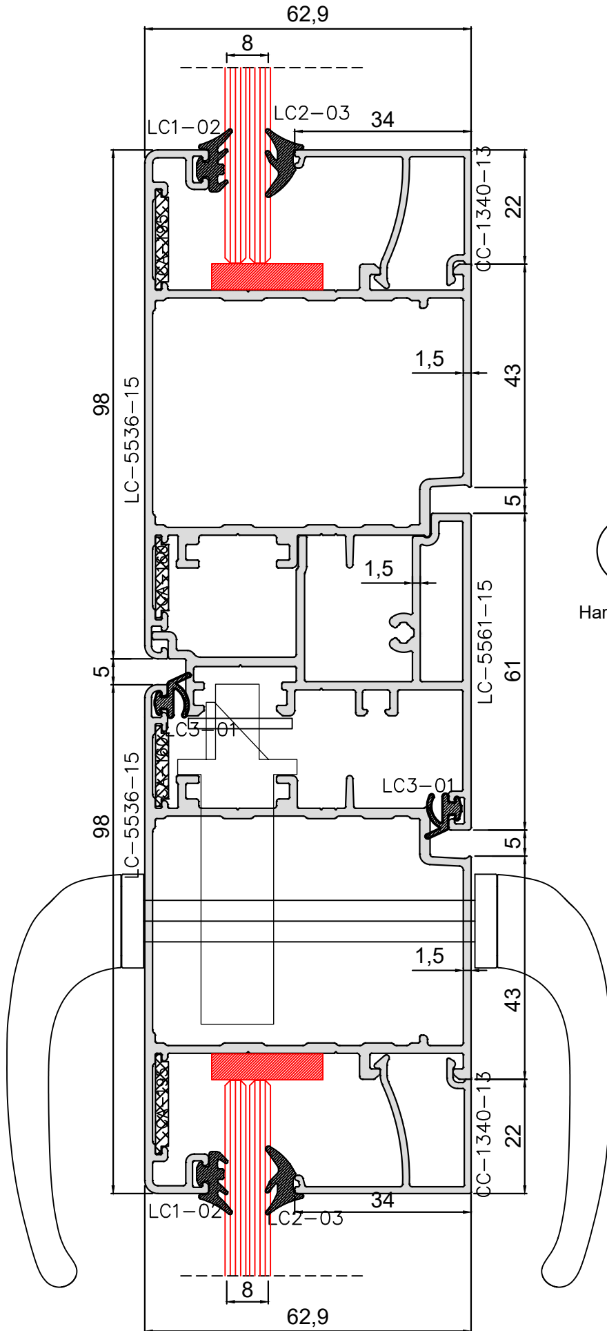
Dışa Açılım Çift KanLC Adaptörü
