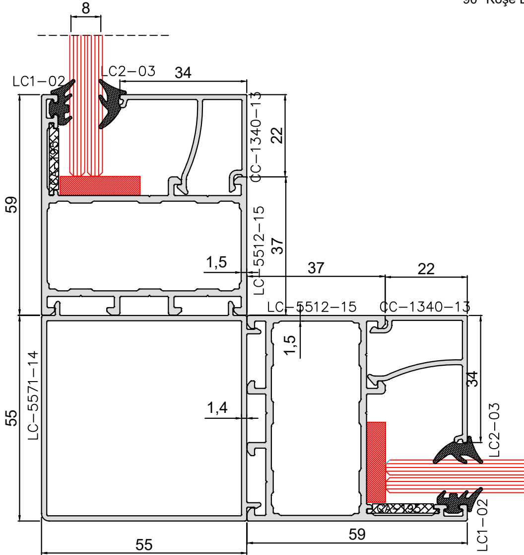
90° Köşe Dönüş
