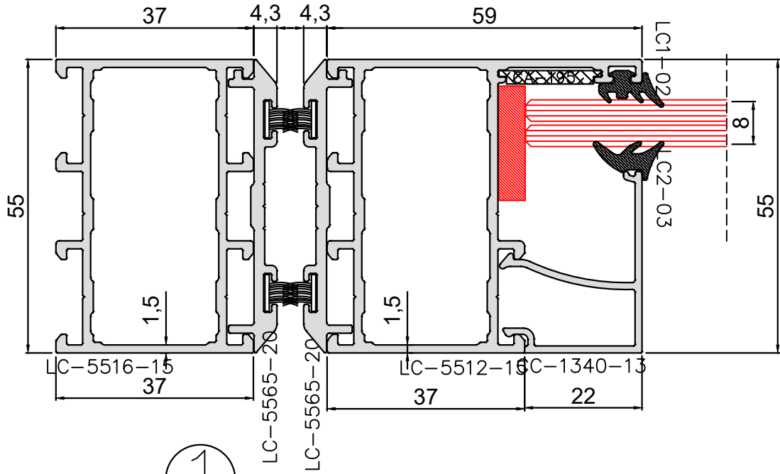
Dar Çarpma Kapı Kasa Detay
