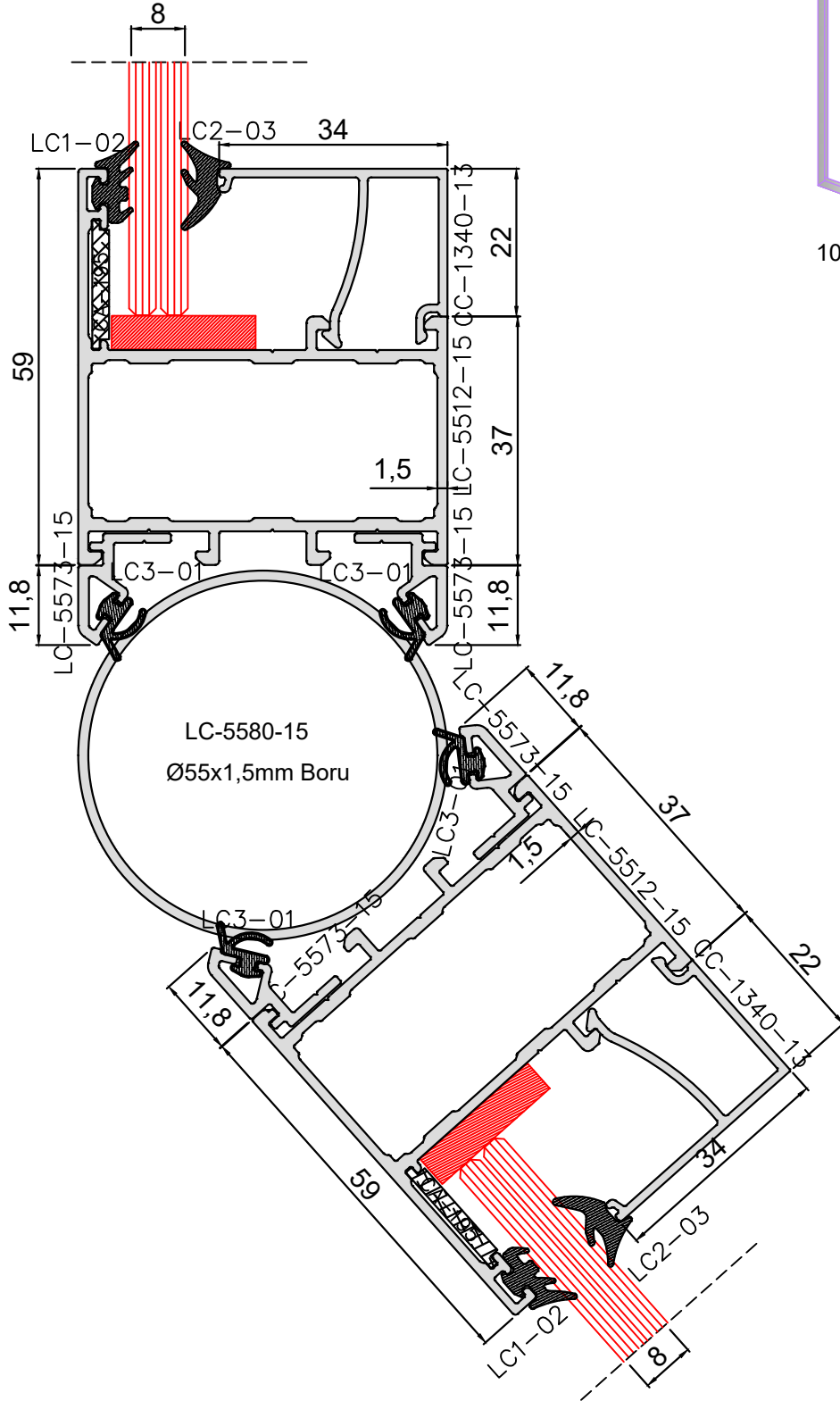
100°-180° Köşe Dönüş Detay
