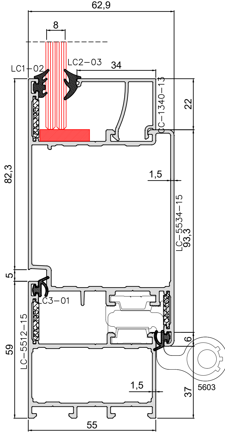
Kapı Menteşe Detay
