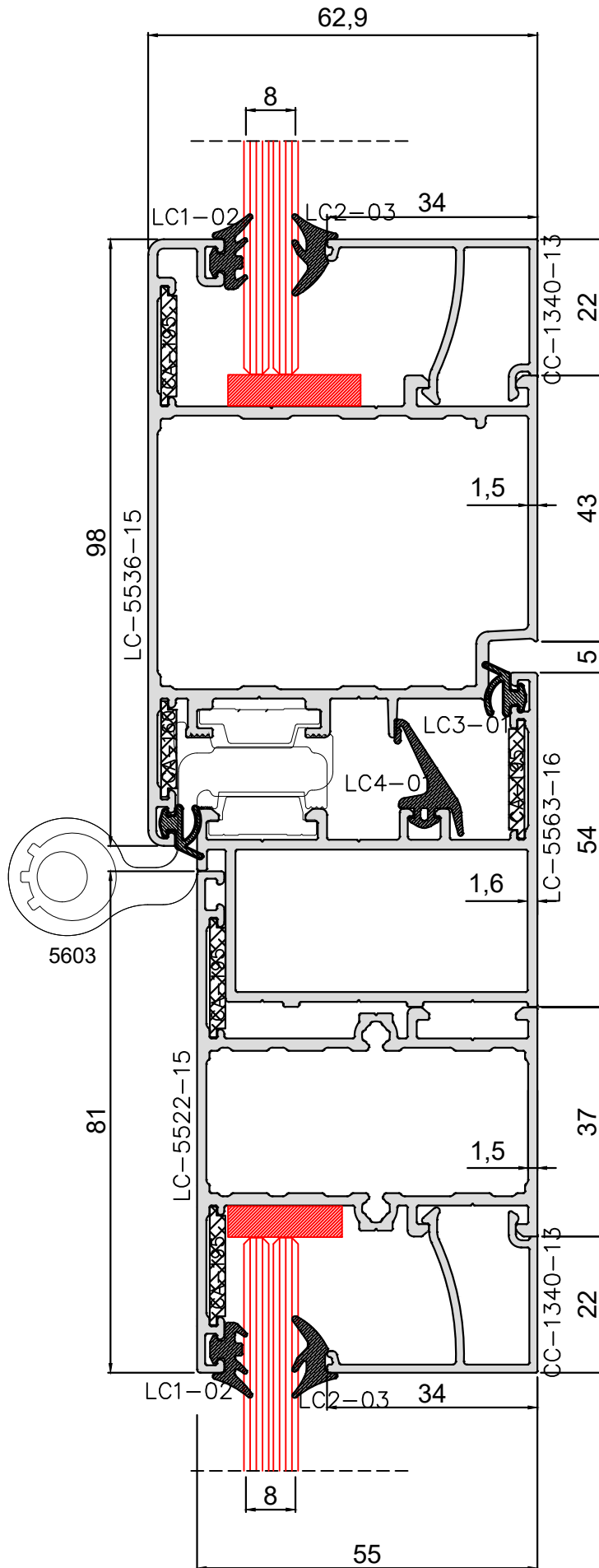
Dışa Açılır Kapı Sabit Detay
