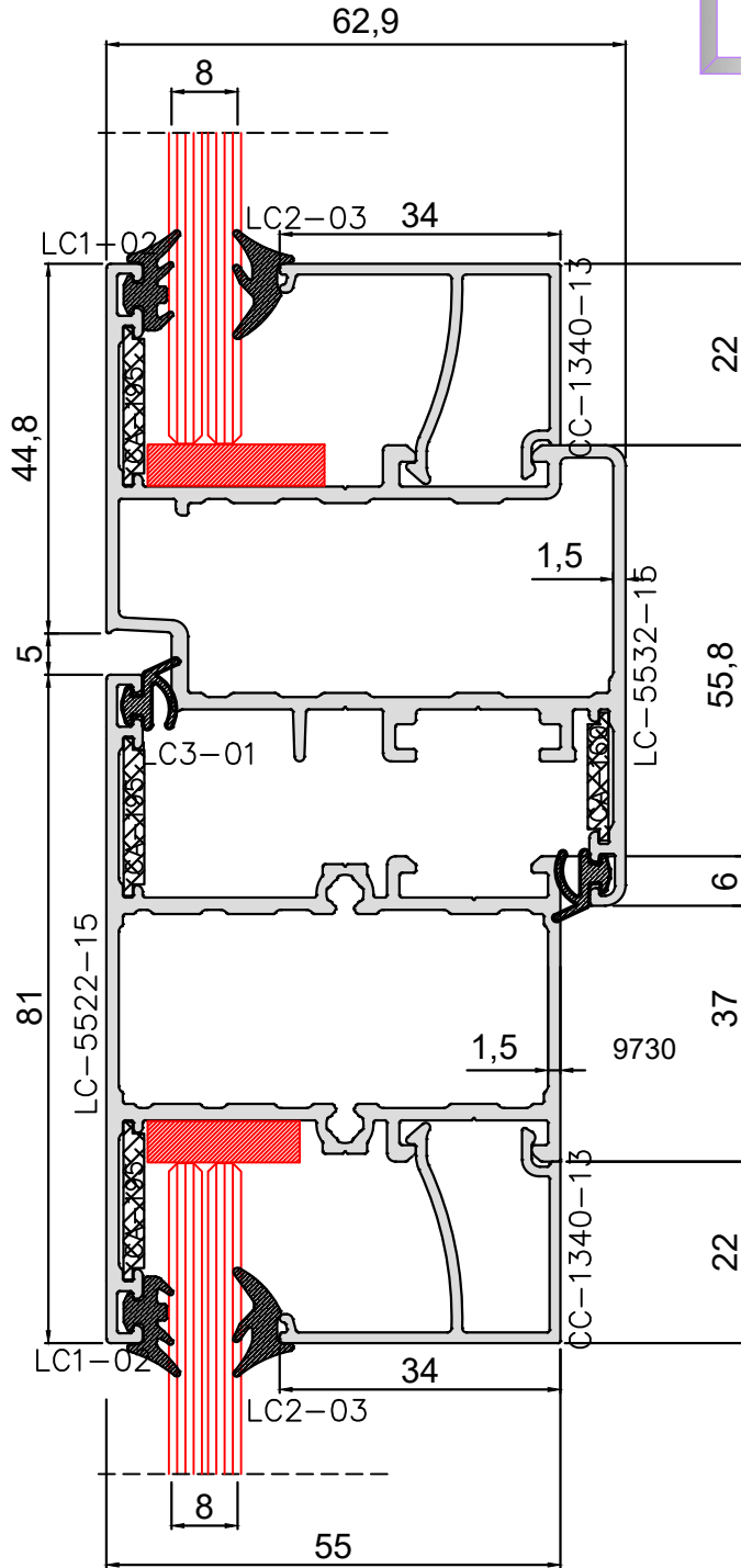
1 Orta Kayıt Açılır Detay
