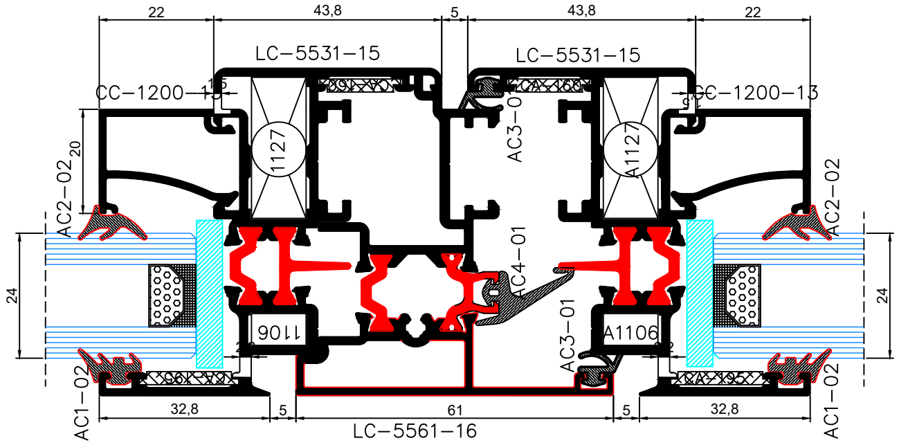
Hareketli Orta Kayıt Açılır Detay
