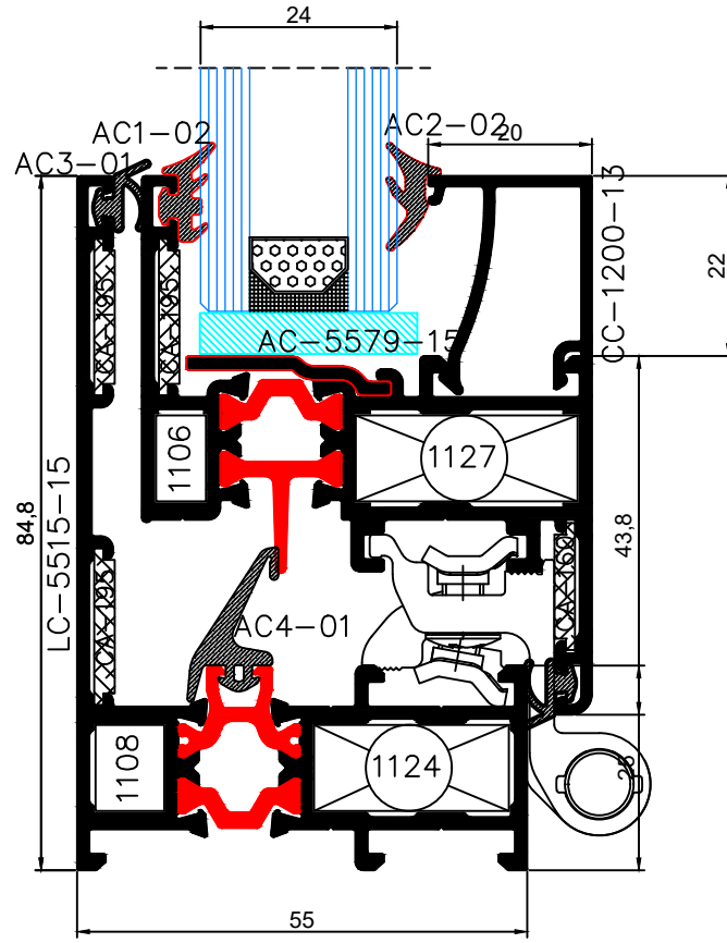
1 Menteşe Detay
