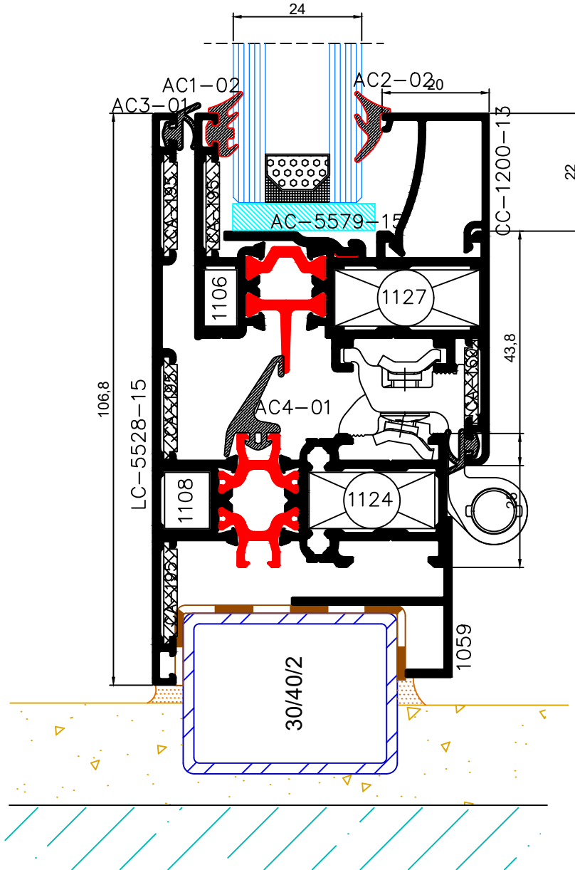
Gizli Kanat Pencere Detayı
