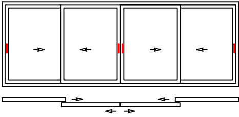
4 HAREKETLİ KANAT 4 SLIDING SASH
